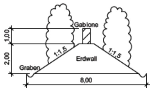
Detailzeichnung: Lärmschutzwall
